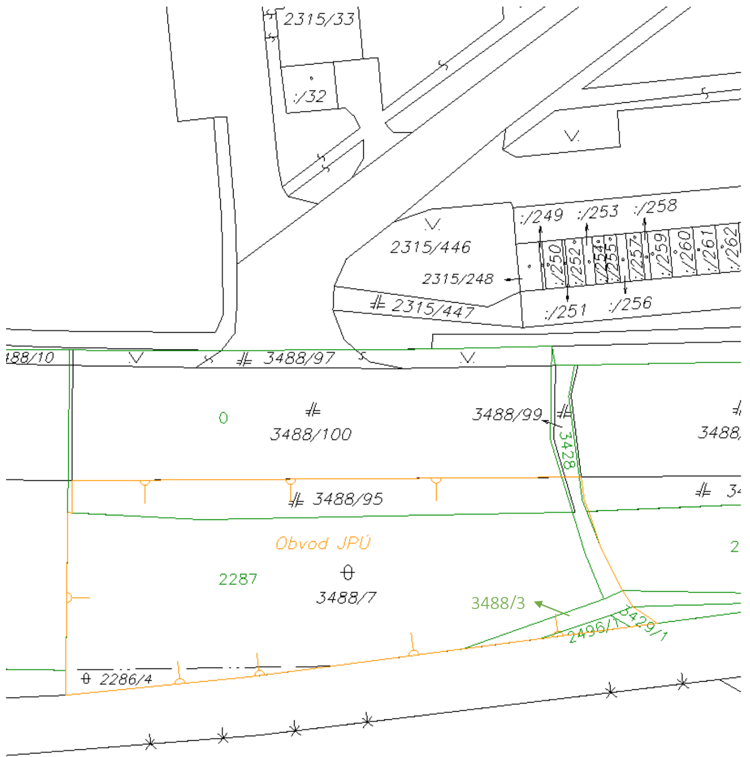
Zákres navrhovaného obvodu projektu pozemkových úprav v časti katastrálneho územia Trenčín, lokalita "CKN p.č. 3488/95 a EKN p.č. 2287"
