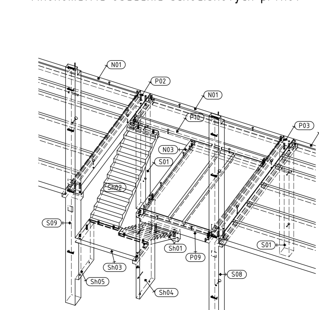
Axonometria osadenia schodiskových prvkov
