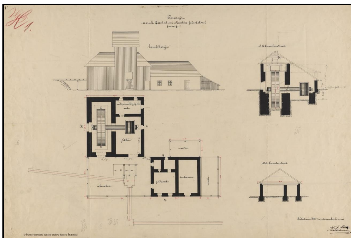
Obr. 1: Budovy šachty Rudolf v ich usporiadaní po prestavbe v roku 1885 s novým ťažným kolesom
