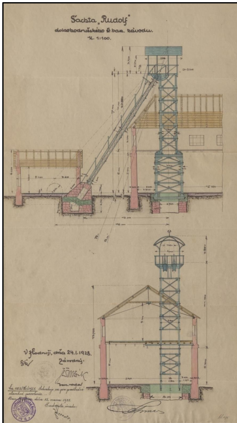
Obr. 3: Nová ťažná veža a šachtová budova so strojovňou na šachte Rudolf v Hodruši, 1928
